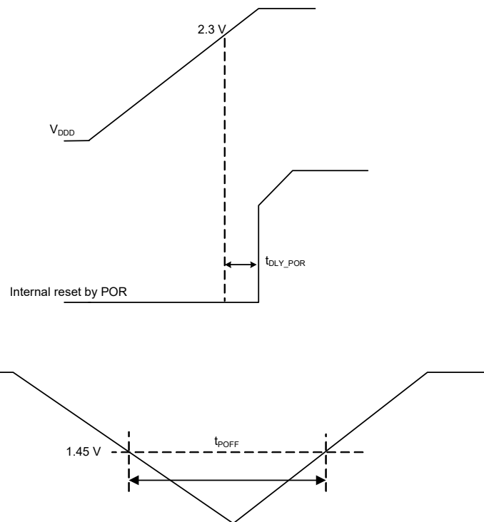
Figure 26-15. POR Specifications
