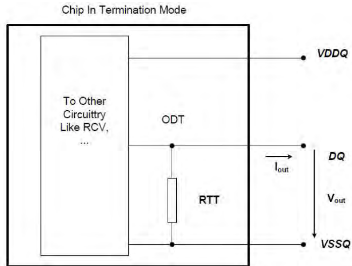
Figure 140 - On Die Termination for DQ
