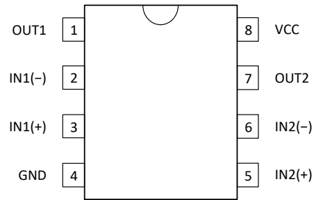
DIP-8
